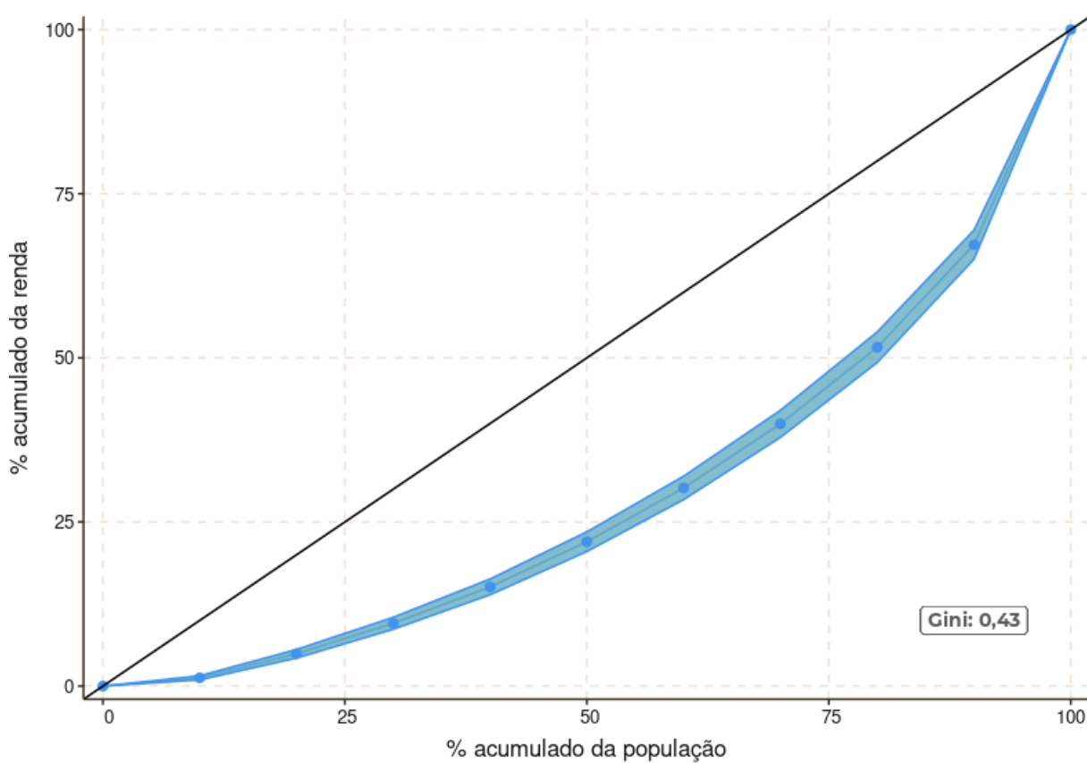
Figura 3.7.4: Curva de Lorenz do rendimento domiciliar, Paranoá, 2021
