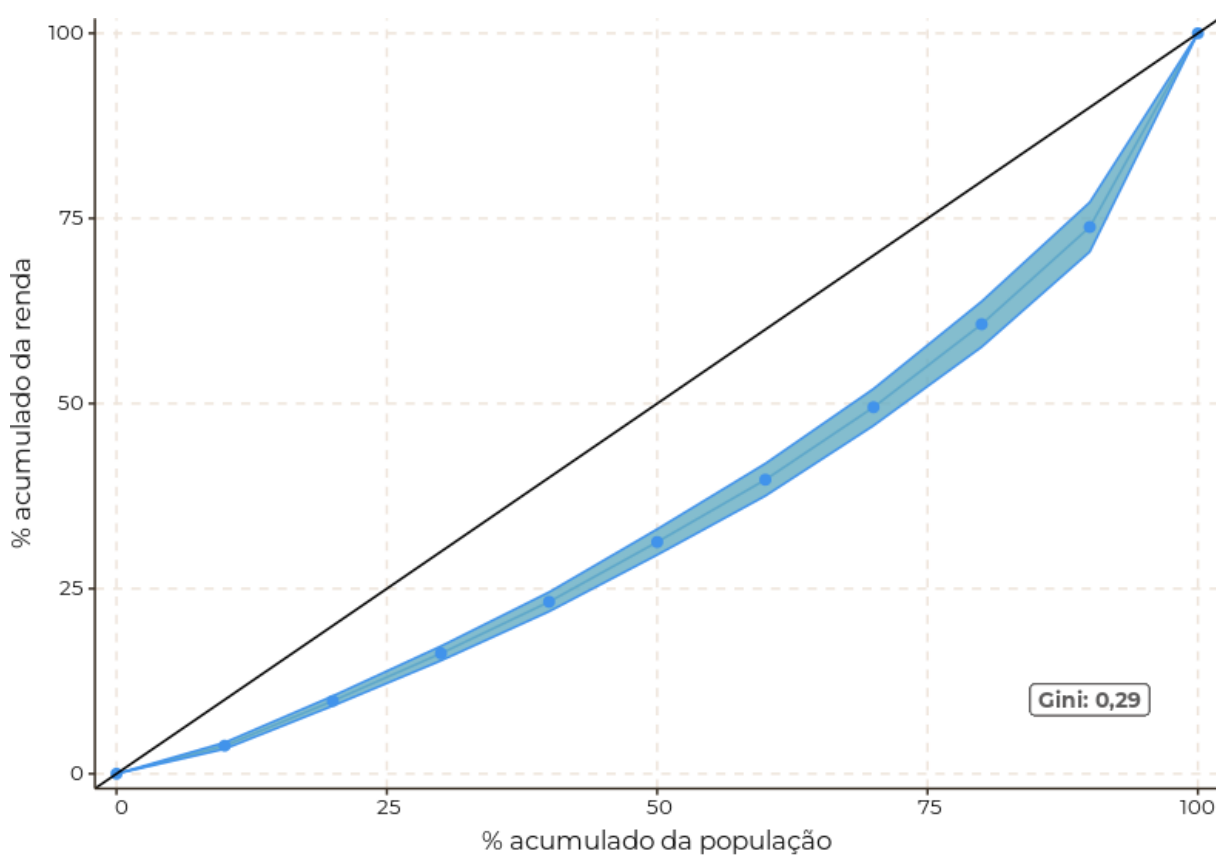
Figura 3.7.2: Curva de Lorenz do rendimento bruto do trabalho principal, Paranoá, 2021
