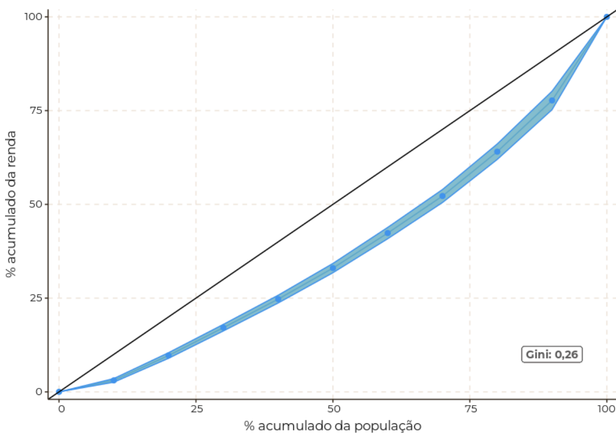
Figura 3.7.2: Curva de Lorenz do rendimento bruto do trabalho principal, Sol Nascente/Pôr do Sol, 2021
