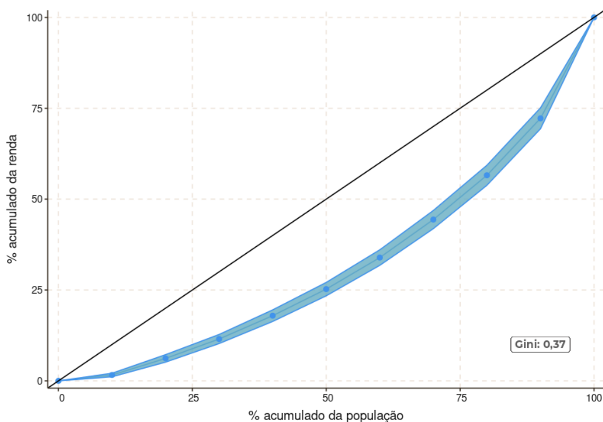
Figura 3.7.4: Curva de Lorenz do rendimento domiciliar, Sol Nascente/Pôr do Sol, 2021
